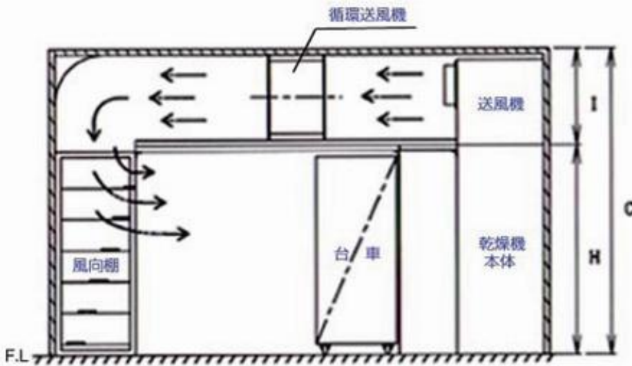
乾燥室 断面図
