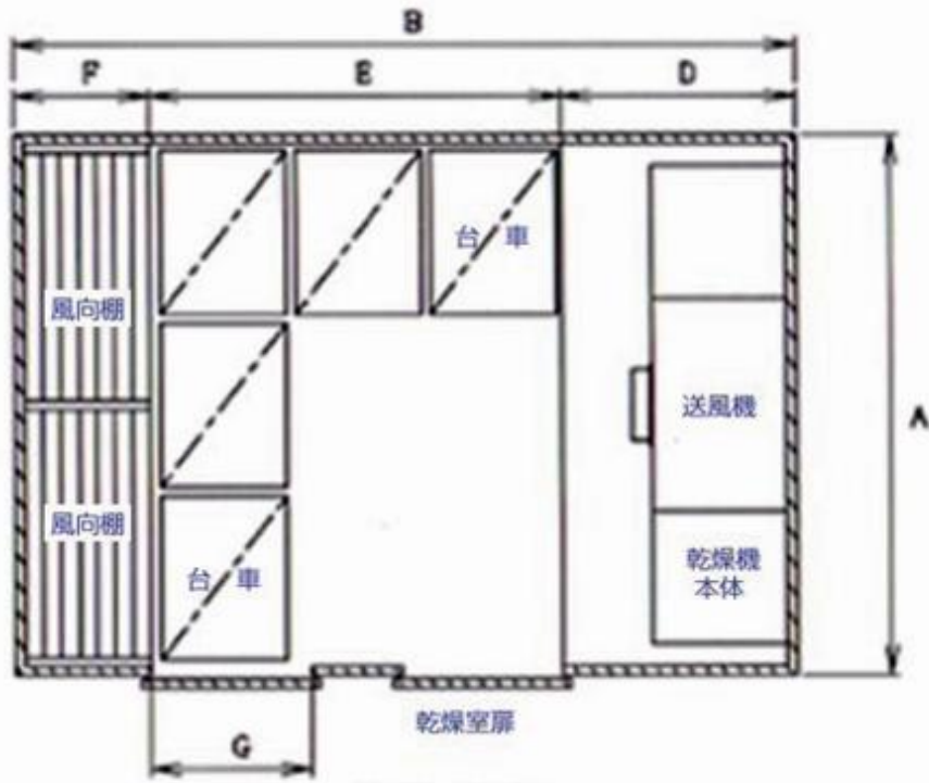
乾燥室 平面図
