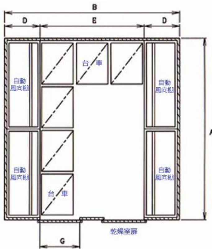
乾燥室 平面図
