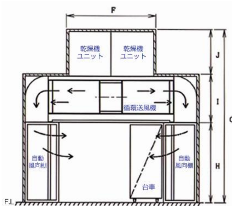
乾燥室 断面図
